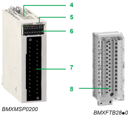
BMXFTB2800
